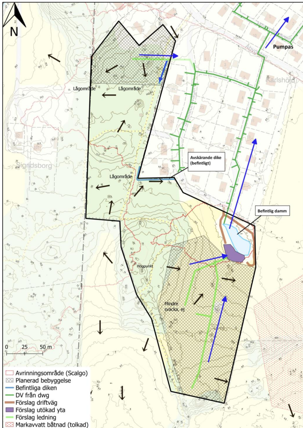
Figur 8. Förslag på framtida dagvattenhantering.
